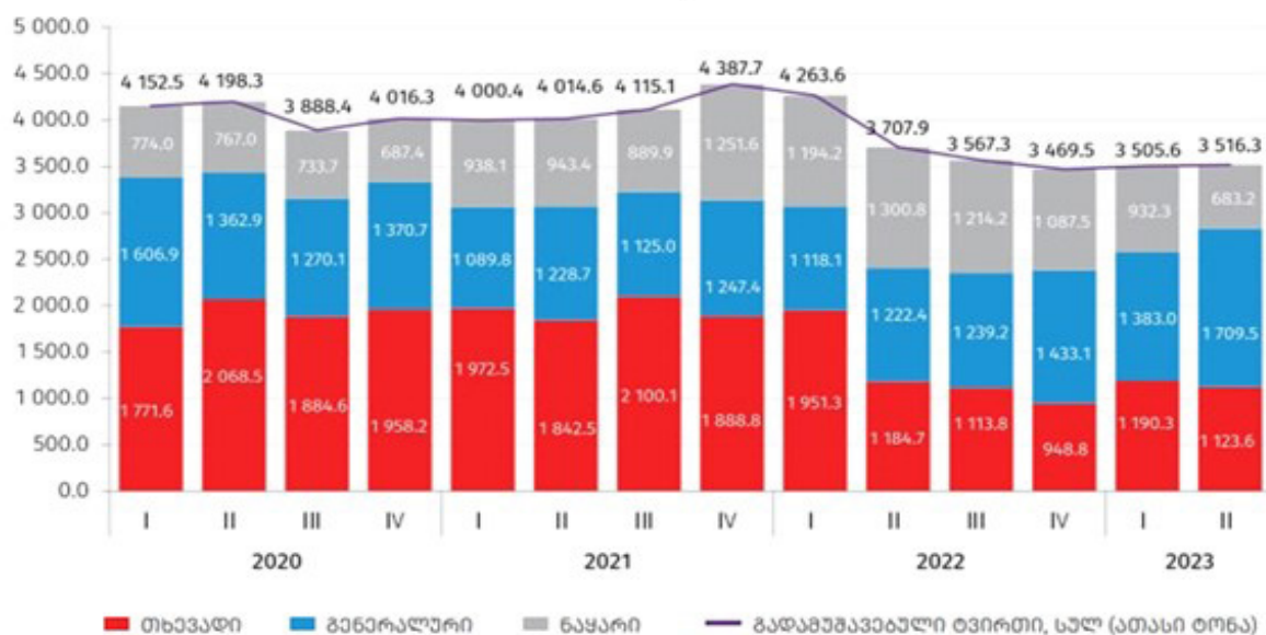
საქართველოს ნავსადგურებში და ტერიტორიაში გადამუშავებული ტვირთის მოცულობა სახეების მიხედვით, ათასი ტონა
